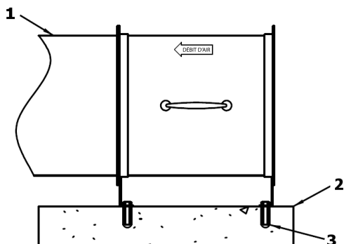
Figure 1. Ventilateur monté sur dalle (ventilateur axial)
